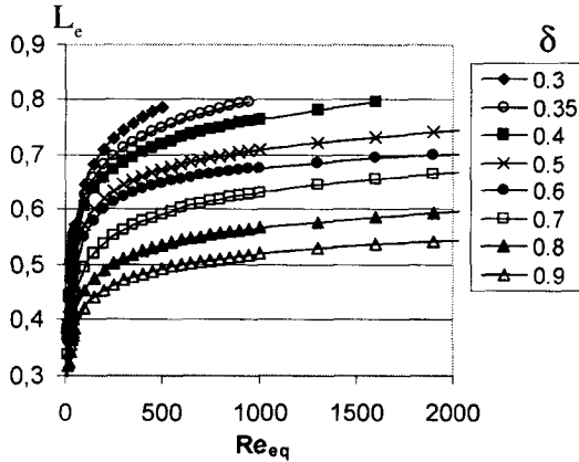
Figure 1. Longueur d'entrée adimensionnelle en fonction du nombre de Reynolds équivalent, pour différentes valeurs du degré de sténose.
