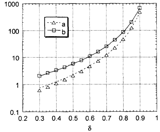
Figure 2. Coefficients a et b (voir § 4) en fonction du degré de sténose. Points : résultats de l'analyse de régression portant sur Re_{eq} à degré de sténose donné. Courbes : résultats de l'analyse de régression finale portant sur le degré de sténose.
